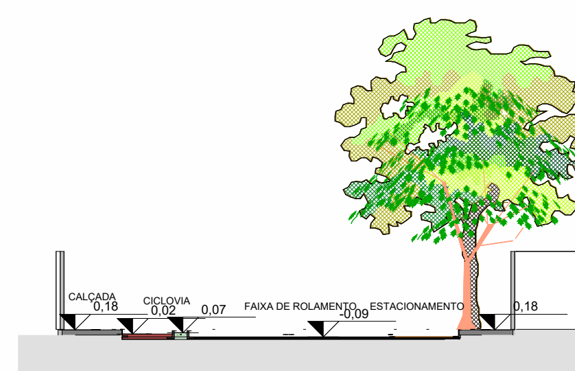
6 PERFIL 04 F03 1 : 200
