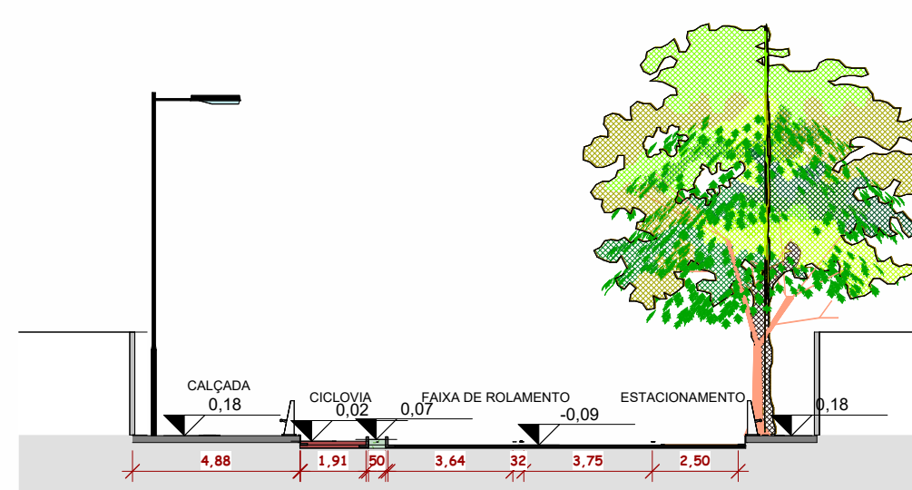
4 PERFIL 02 F03 1 : 200
