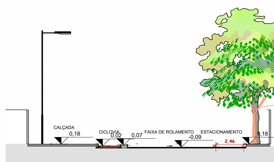
5 PERFIL 03 F03 1 : 200
