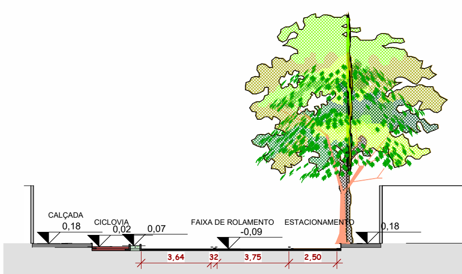
3 PERFIL 01 F03 1 : 200
