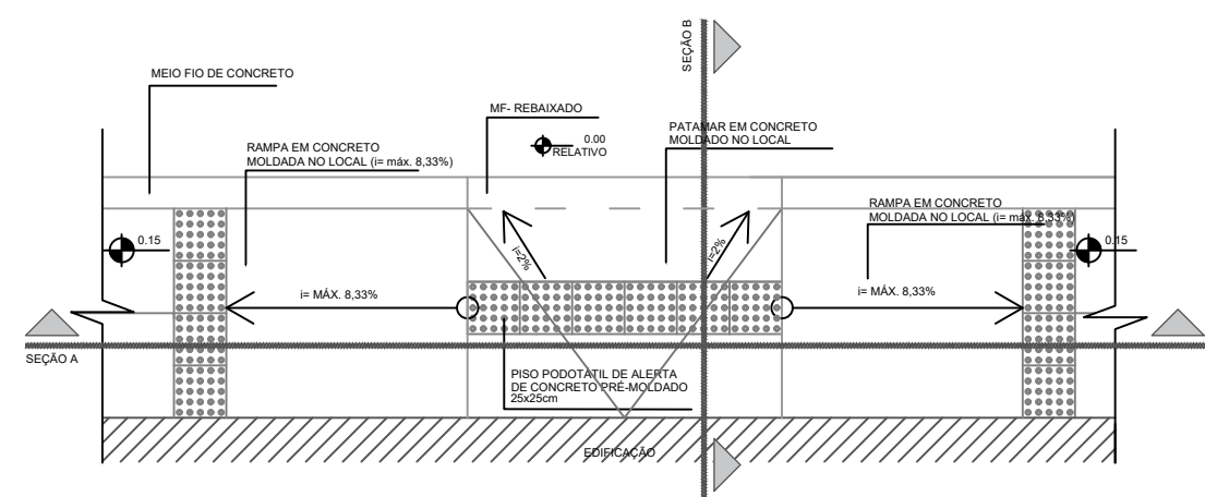
- DETALHE DA RAMPA S/ ESCALA
