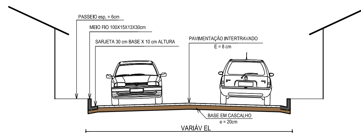
PERFIL TRANSVERSAL SEM CONTENÇÃO CORTE - BB S/ ESCALA
