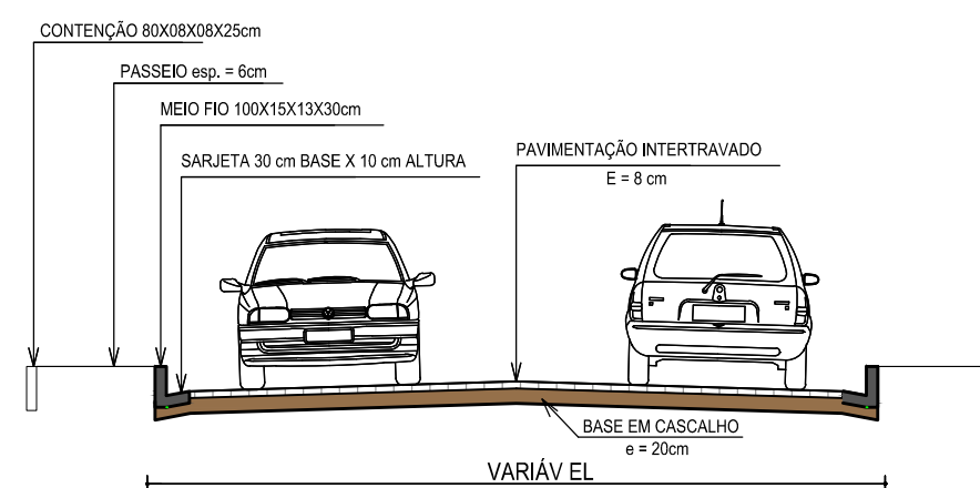
PERFIL TRANSVERSAL COM CONTENÇÃO CORTE - BB S/ ESCALA
