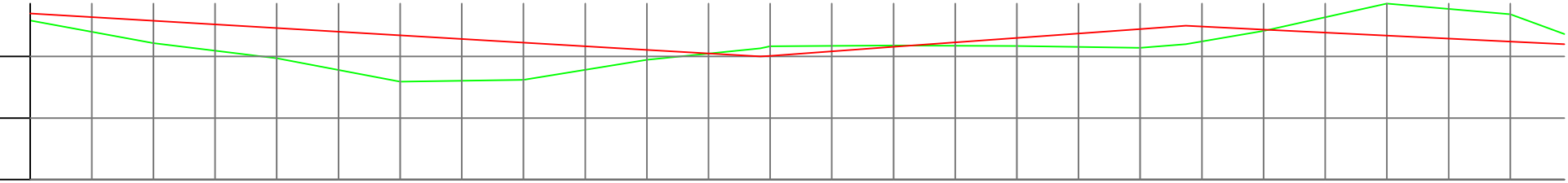
PERFIL LONGITUDINAL ESCALA – H=1/1.000; v=1/100
