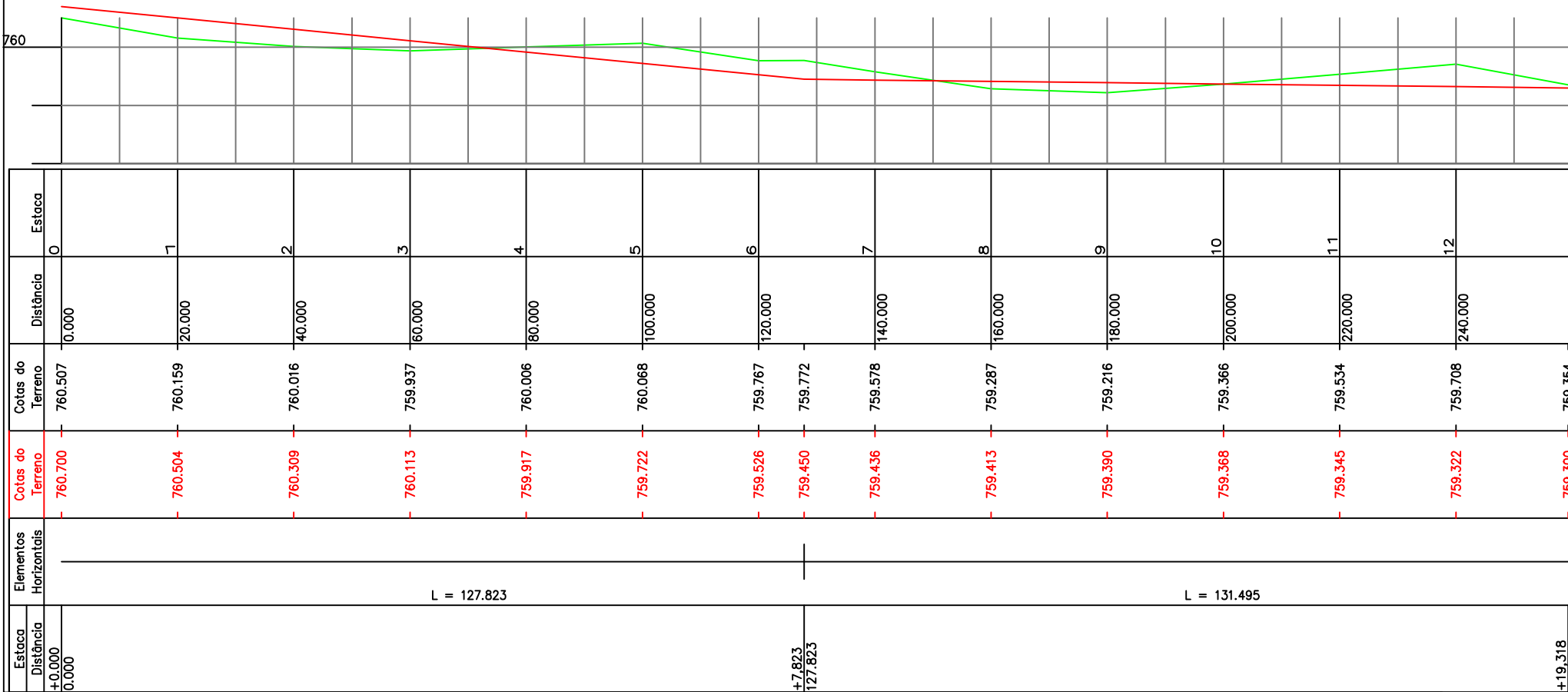
PERFIL LONGITUDINAL ESCALA – H=1/1.000; V=1/100
